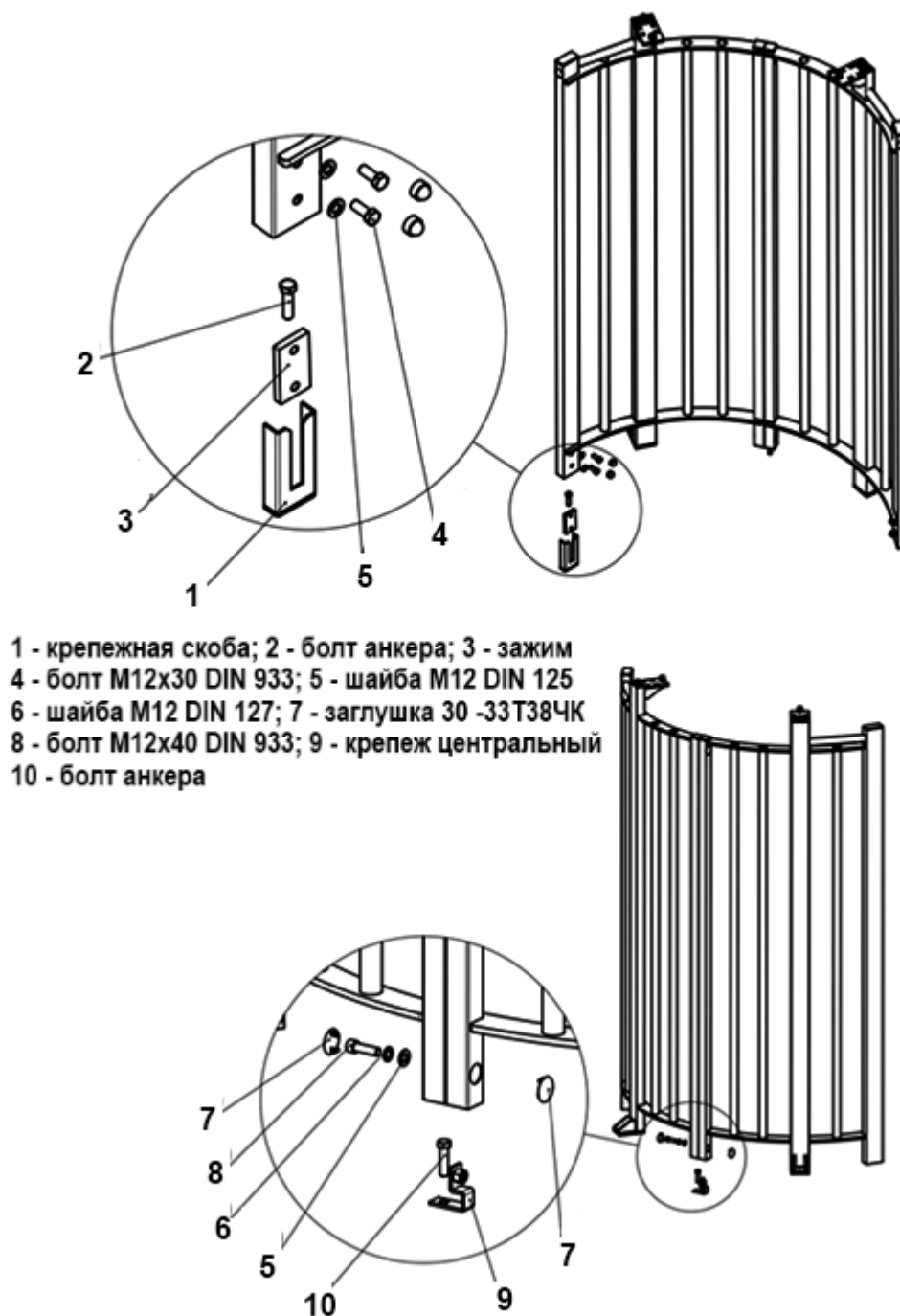
Рисунок 7 – Крепление неподвижной панели ограждения
