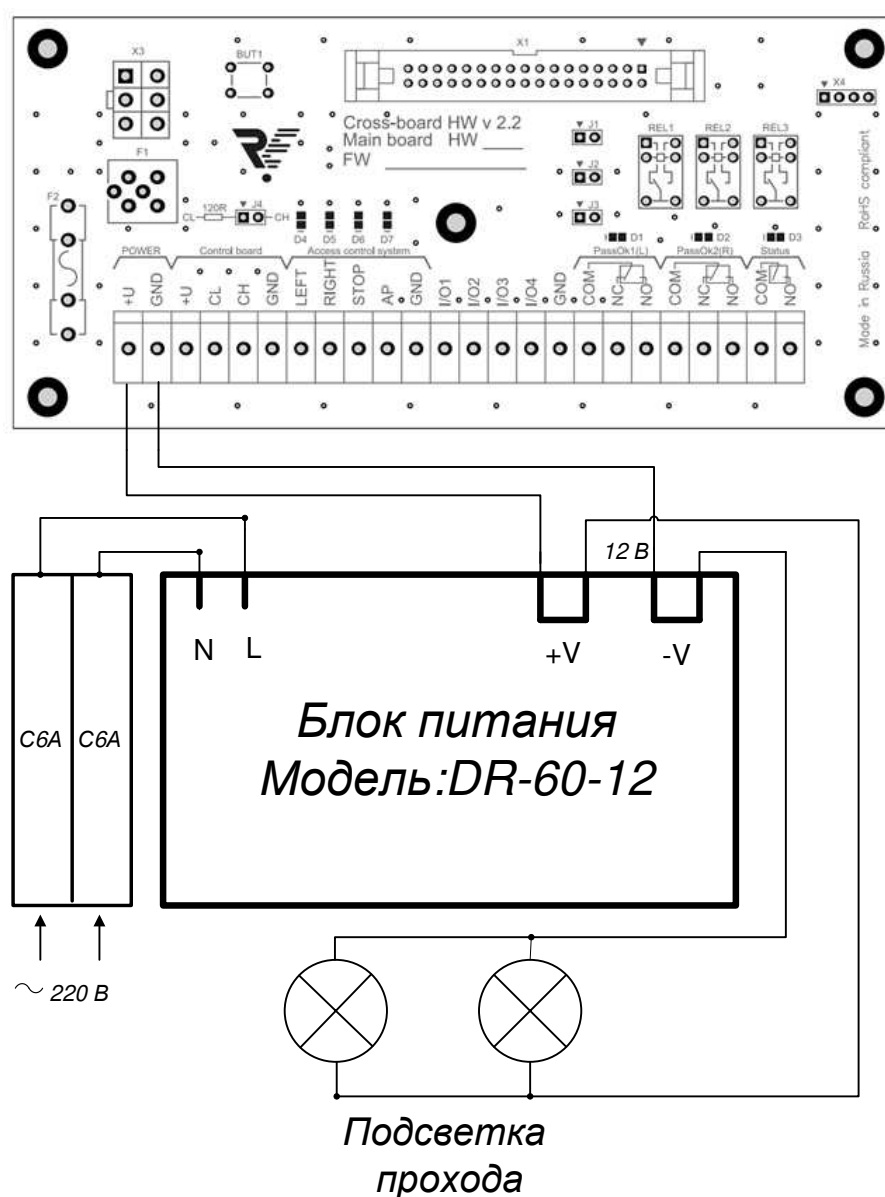
Рисунок 14 – Схема подключения питания турникета
