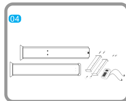
04 Подготовьте антенные панели, электронный блок, перекладны и крепежные винты.
